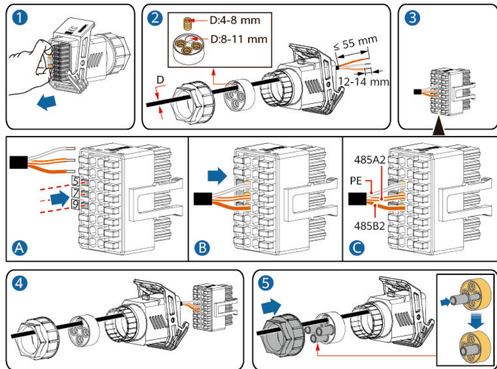
Abbildung 5-25 Kabelmontage
