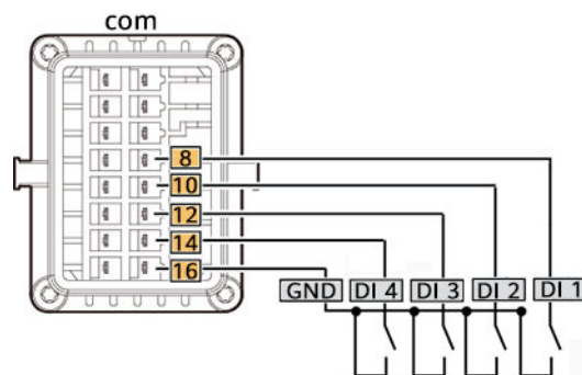
Abbildung 5-29 Kabelverbindung
