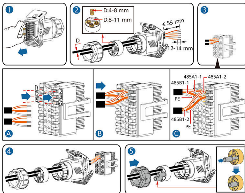
Abbildung 5-21 Kabelmontage
